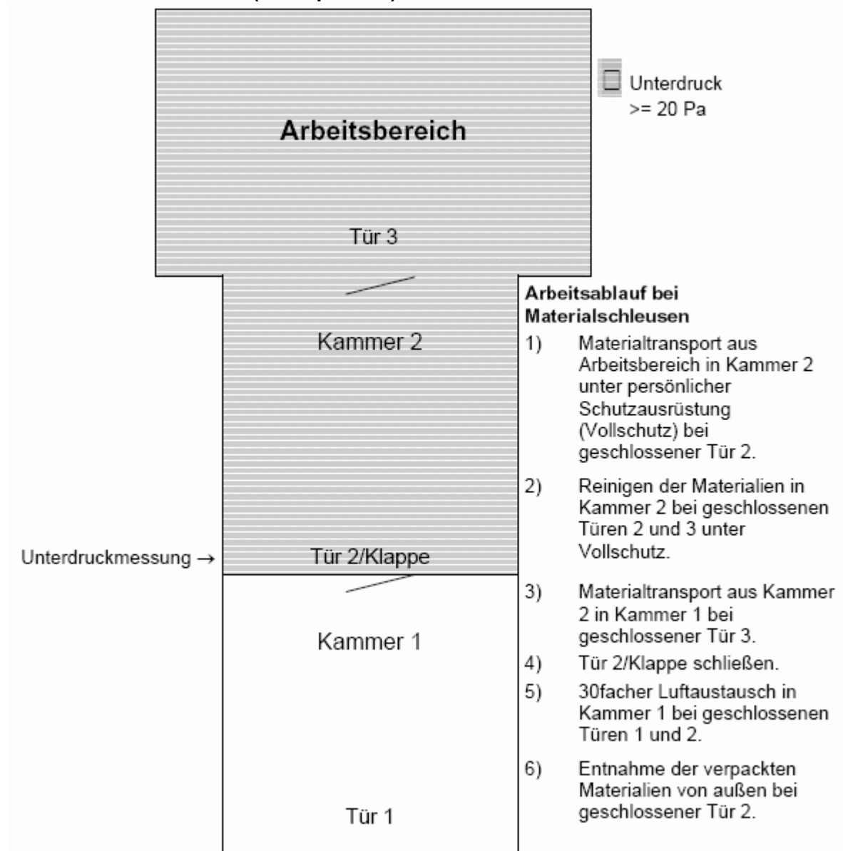
Abb. 2 Materialschleuse (Prinzipskizze)
