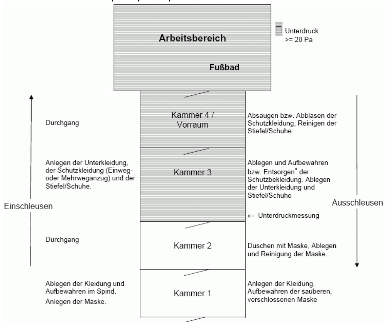
Abb. 1 Personenschleuse (Prinzipskizze)
